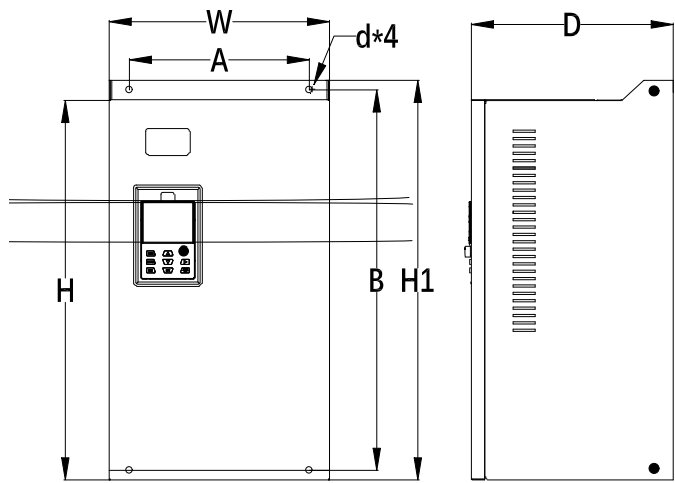
205~212 钣金机箱代码示意图
