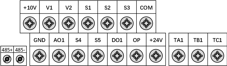
101/102 系列机箱接线端子
