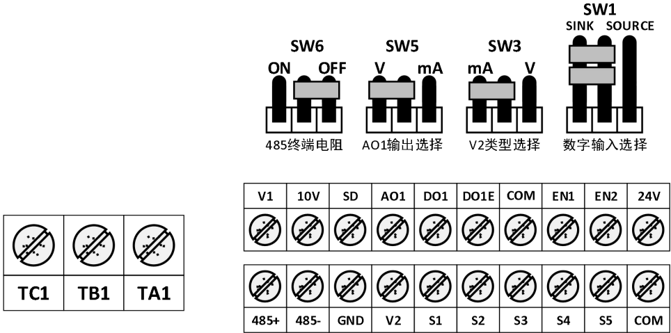
201/202 系列机箱接线端子
