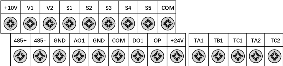
103/208 ~ 215 系列机箱接线端子
